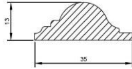
Sez. A-A
